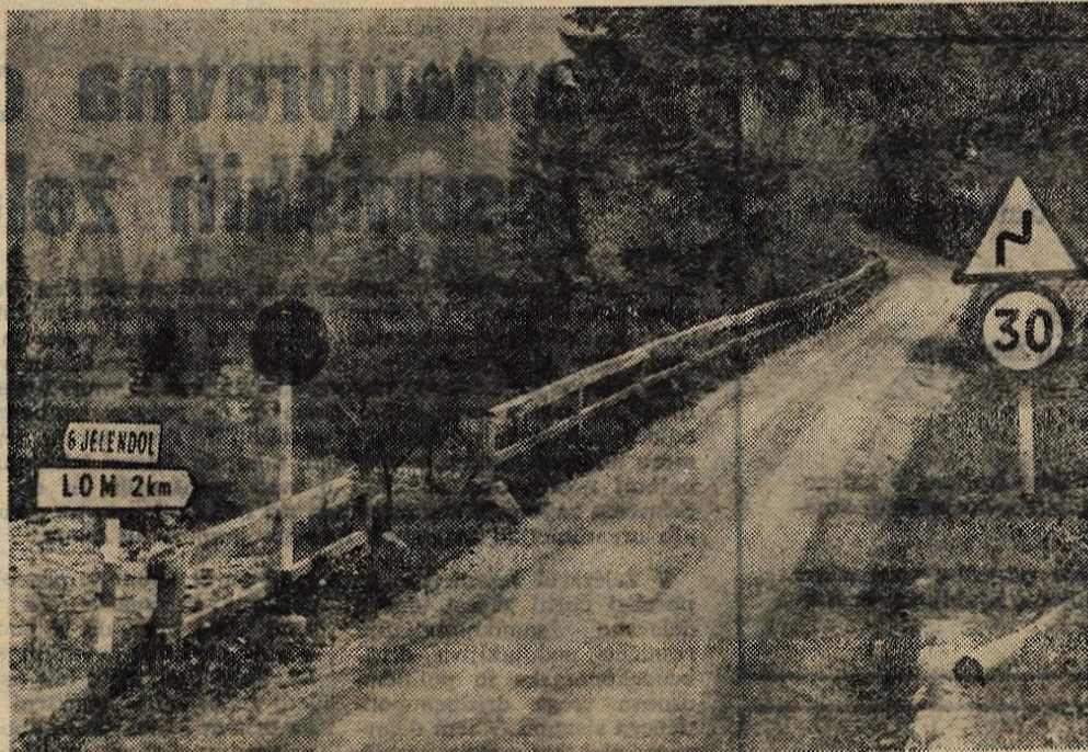
Ozko grlo na sedanji cesti v Lom je tudi klanec takoj po priložu iz Tržiča. Nova cesta, ki jo nameravajo graditi, takih strmih vzponov ne bo imela, saj bo potekala po položnejšem zemljišču. (Jk) — Foto: F. Perdan
