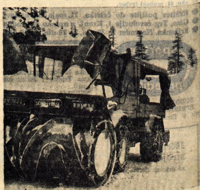
Snežni stroji VF-3 so sposobni premagati tudi največje plazove. Uporabljajo jih že po vseh alpskih državah Evrope.
