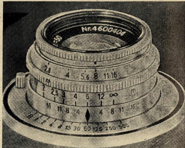
Objektiv fotoaparata Werra. Zgornje oznake predstavljajo zaslonke od 2,8 do 16. V sredini imate oznake za metre. Vidijo se le od 1,7 pa do neskončno. Aparat ima najmanjšo razdaljo od 0,9 metra. Pod metražo imate ponovno zaslonke, s katerimi lahko približno določite globinske interval ostrine, in sicer je pri zaslonki pri isti razdalji 6 m in 4 ostro od 4,5 pa vse do 12 metrov. Pri zaslonki 8 pa že od 3,5 in skoraj do neskončnega, pri zaslonki 11 pa že od 2,8 do neskončno. Spodaj imate še čase, in sicer: B, 1 sekunda, 1/2 sek., 1/4 sek., 1/8 sek., 1/15 sek., 1/30 sek., 1/60 sek., 1/125 sek., 1/250 in 1/500
