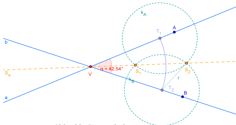
Slika 38: Simetrala kota
