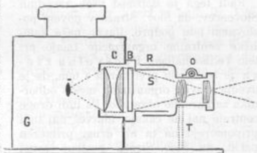
Sestavni deli skioptikona.
