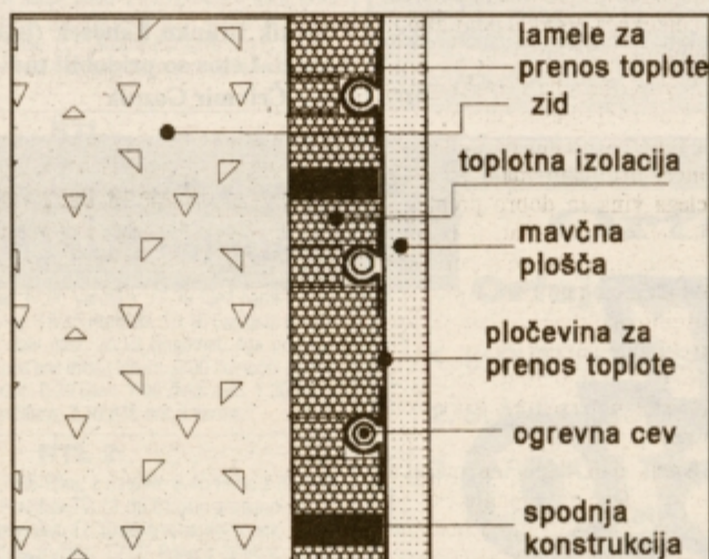
Stensko ogrevanje s površinsko nameščenim cevnim sistemom pod ometom - suh način vgradnje
