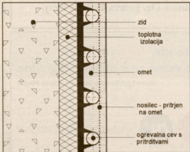
Stensko ogrevanje s površinsko nameščenim cevnim sistemom pod ometom - moker način vgradnje
