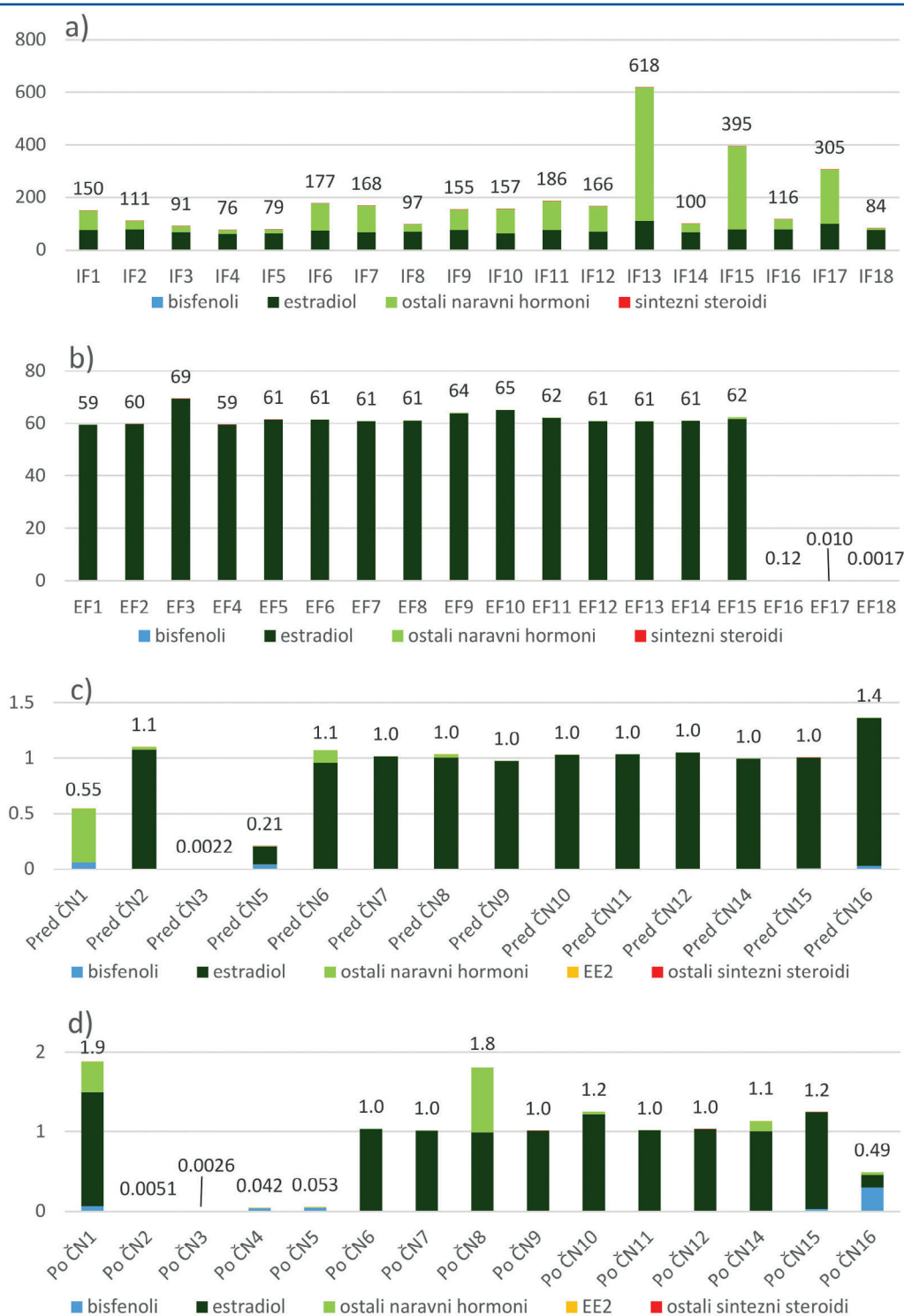
Slika 2: Skupni estradiolski ekvivalenti v ng/L po izbranih spojinah (na y osi) in skupinah v a) vtokih čistilnih naprav, b) iztokih čistilnih naprav in vzorcih rečnih vod, odvzetih c) pred in d) za čistilnimi napravami v posameznih vzorcih (x os).
