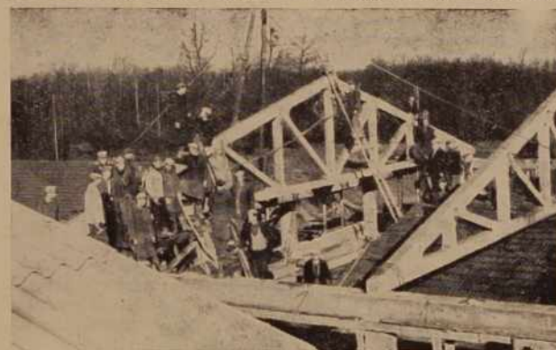
Montaža strešnih nosilcev v opekarni Lukavci, ki jo je opravilo Gradbeno podjetje Gornja Radgona
