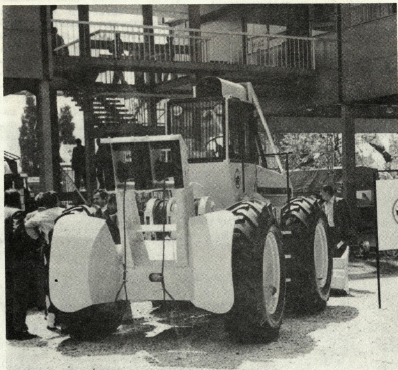
Pogled na zgibnik IMT 5131 z zadnje strani. Foto: Šolar Z.
