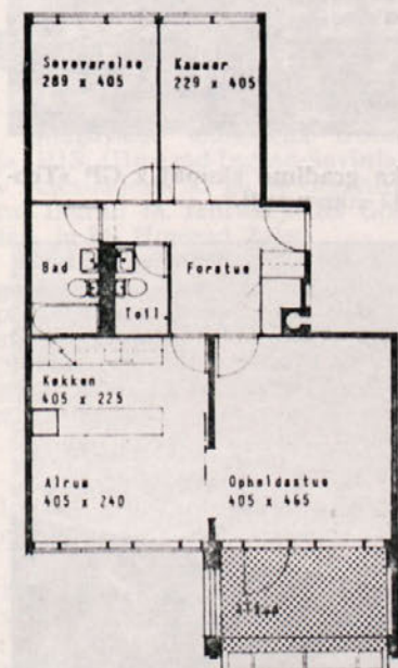
Tloris dvoipol-sobnega stanovanja s površino 97 m 2 . Viden je instalacijski voz, ki združuje sanitarije in kuhinjo v skupno vertikalno
