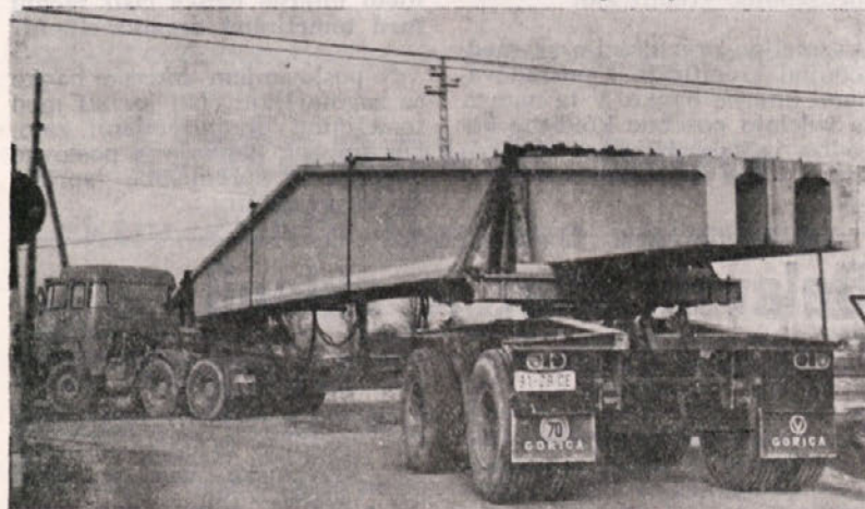
Prevoz montažnih elementov za hale
