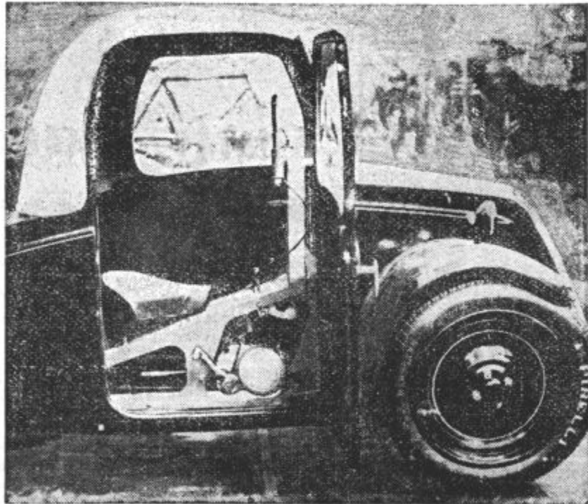
MOTOCIKEL S TREMI KOLESI. Ta motocikel s tremi kolesi napravlja vtis malega avtomobila. Vrhu tega je zelo poceni, ker ne rabi močnih cilindrov.
