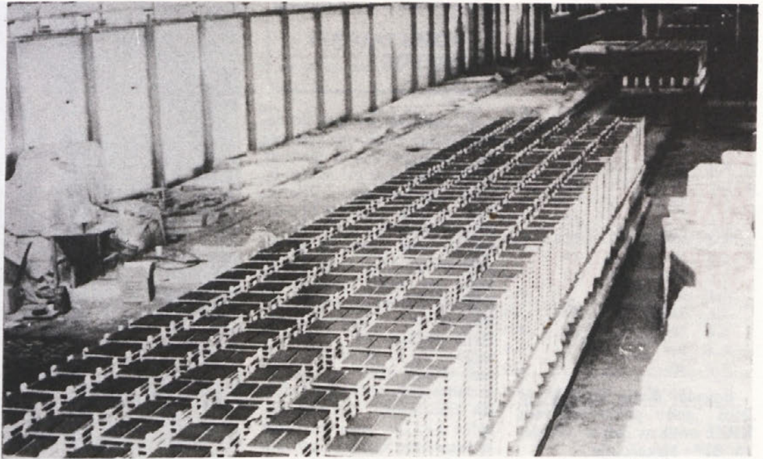
Več tisoč keramičnih ploščic, ki so pravkar zapustile peč se počasi ohlaja. V celotnem proizvodnem procesu pravzaprav sploh ni opaziti delavcev, kar potrjuje, da je celotni postopek visoko avtomatiziran.
