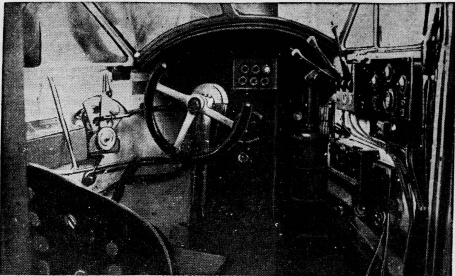
Pogled v pilotov prostor s pripravami za avtomatično stabiliziranje in ravnanje letala. Na levi poleg volana tako zvanega anemometer, ki ureja vzlet, na desni trije vzvodi za stabilizacijo letala v treh ravninah, za volanom pretikalna plošča s gumbi
