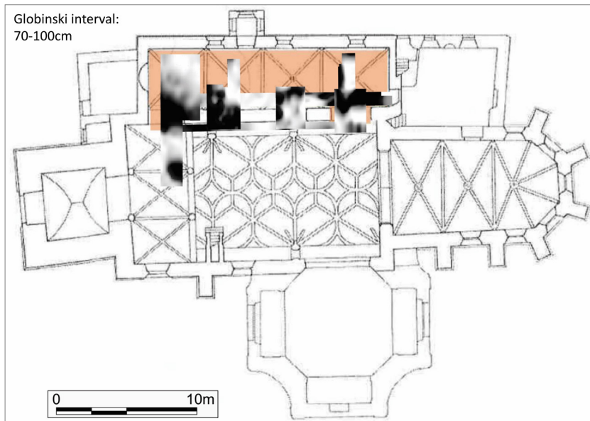
14. Slovenske Konjice, župnijska cerkev sv. Jurija, rezultati prve georadarske meritve na globini 70–100 cm (© Branko Mušič)
