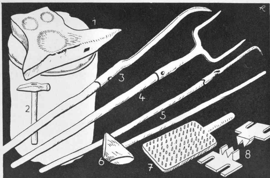
Sl. 2. Nekaj zvončarskega orodja z Višelnice: 1. nakovalo z modli za bokanje zvoncev, 2. kladivo za bokanje zvoncev, 3. »rašpa« za obracanje pušljev na ognju, 4. vile za prenašanje pušljev, 5. »kavka« za valjanje pušljev po tleh, 6. »čij« za tolčenje ilovice, 7. »mašina« za puljenje prediva, 8. klini (»štance«) za urezavanje ploščic (risal I. Romih)
