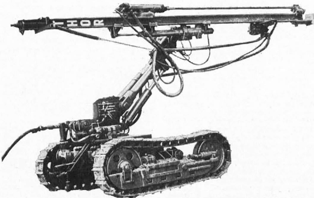
Slika 12 — težki vrtalni stroj na gosenicah (tuja izdelava). Vsi premiki se opravljajo prek cilindrov na hidravlični pogon
