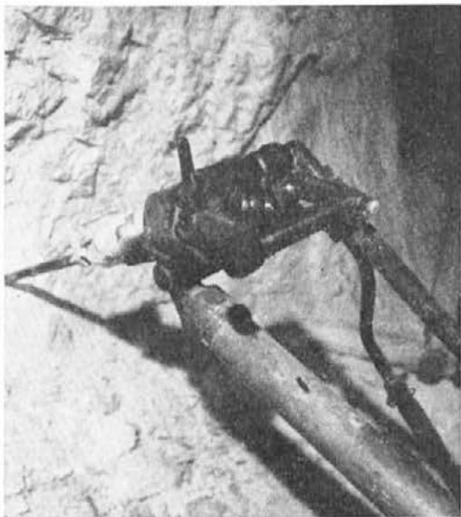
Slika 3 — najnovejši izdelek; 28-kg kladivo s centralno komando na glavi in povratno podporno nogo
