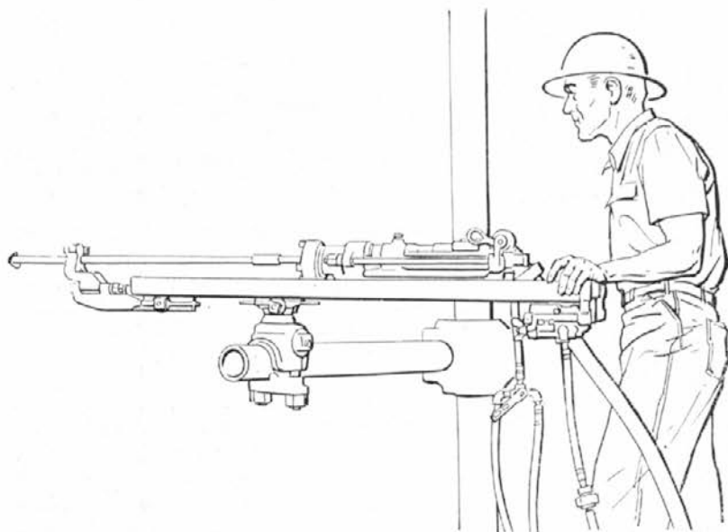
Slika 1 — vrtanje s starimi težkimi stroji na stebrih
