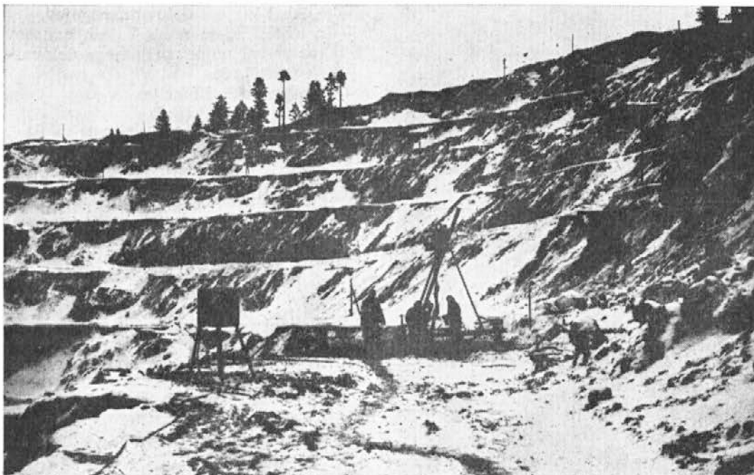
Slika 11c — globinski vrtalni stroj Ravne na etažah rudnika železne rude Vareš
