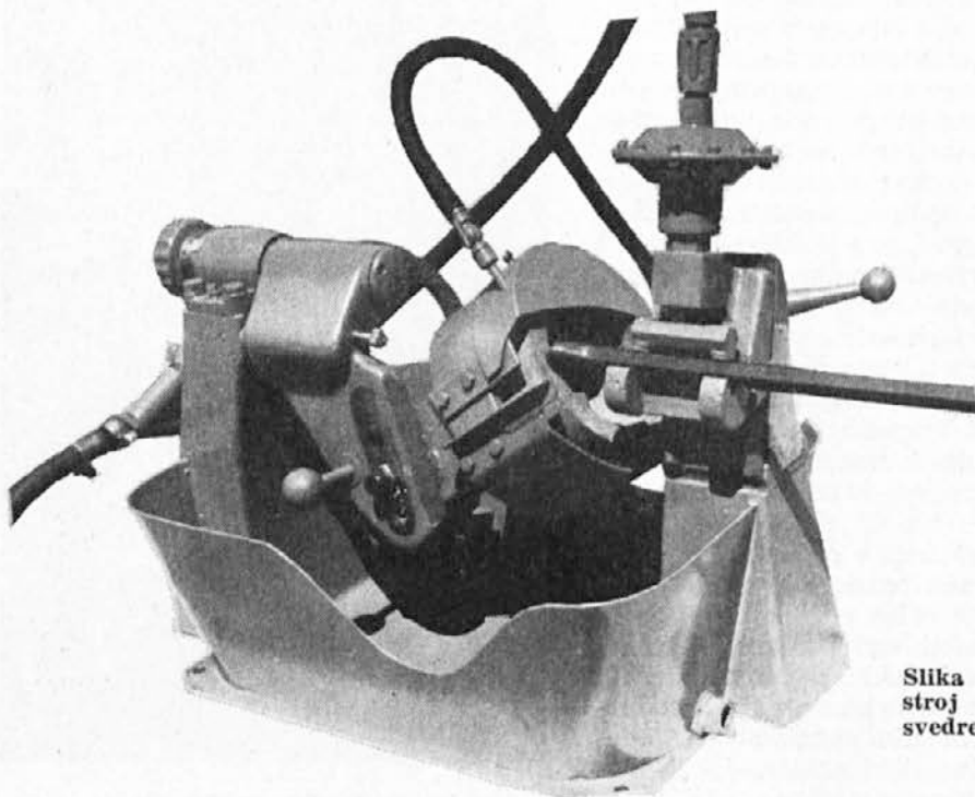
Slika 11 a — globinski vrtnalni stroj na kamnolomu Pirešica
