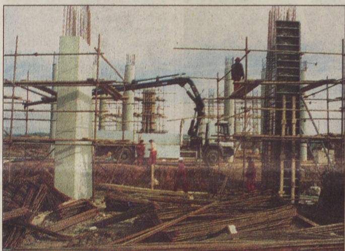
Premostitveni objekti napovedujejo začetek gradnje AC pri nas. (FOTO: N. JUHNOV)
