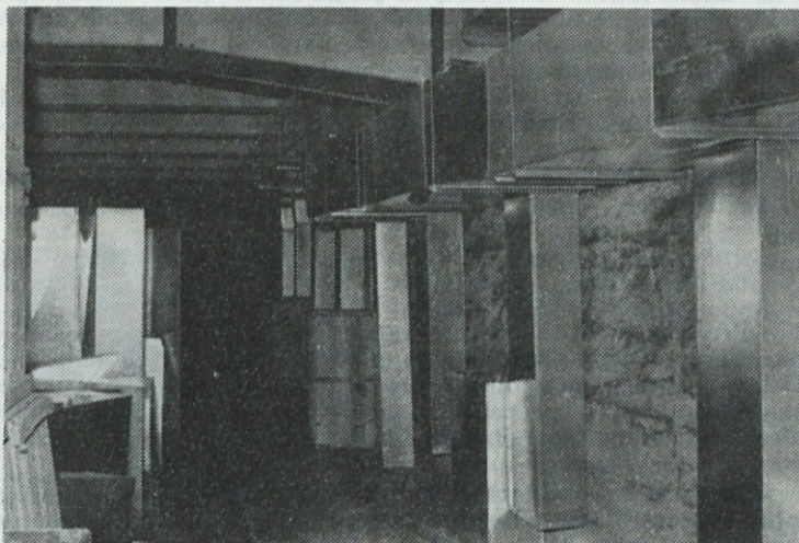
Nameščanje klimatskih naprav v novi predilnici za brezvretensko predenje
