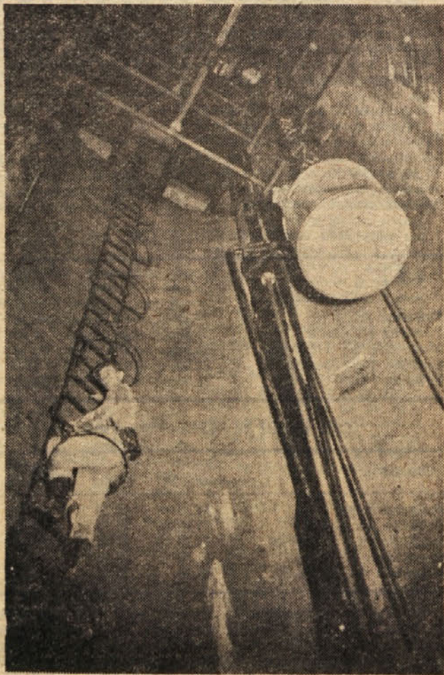
Vzhodni del jaška za visečega jadra v Rudniku lignita Velenje. Izvajalec: Obrat za specialna rudarska dela Rudnika Trbovlje — Hrastnik
