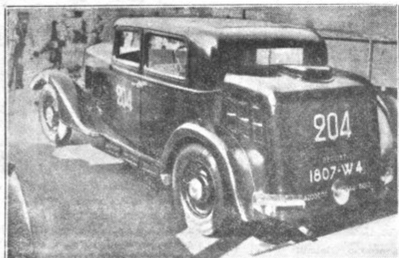
OD BENCINA K LESU. Potniški avtomobil na pogon z lesnim plinom: vplinjevalec je nameščen na zadnjem delu voza
