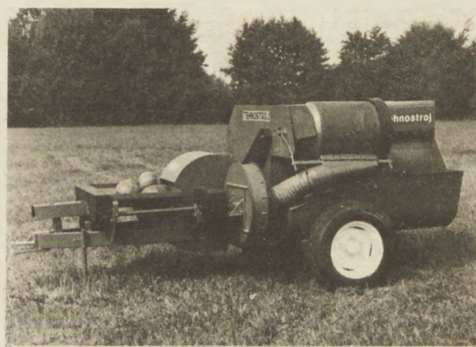
Stroj za luščenje buč (dodali pa mu bodo še stroj za pranje semena) bo v maloprodaji v začetku prihodnjega leta za okrog 5 milijonov dinarjev, razvili so ga strokovnjaki Tehnostrojeve razvojne službe. To je eden v množici primerov, ki so neoporek dokaz strategije premagovanja poukrepnih težav, obenem pa gre za sodobno trženjsko nastopanje s kakovostnimi stroji. Tak način mora tudi v takomimovani dogovorni ekonomiji obroditi sadove.
