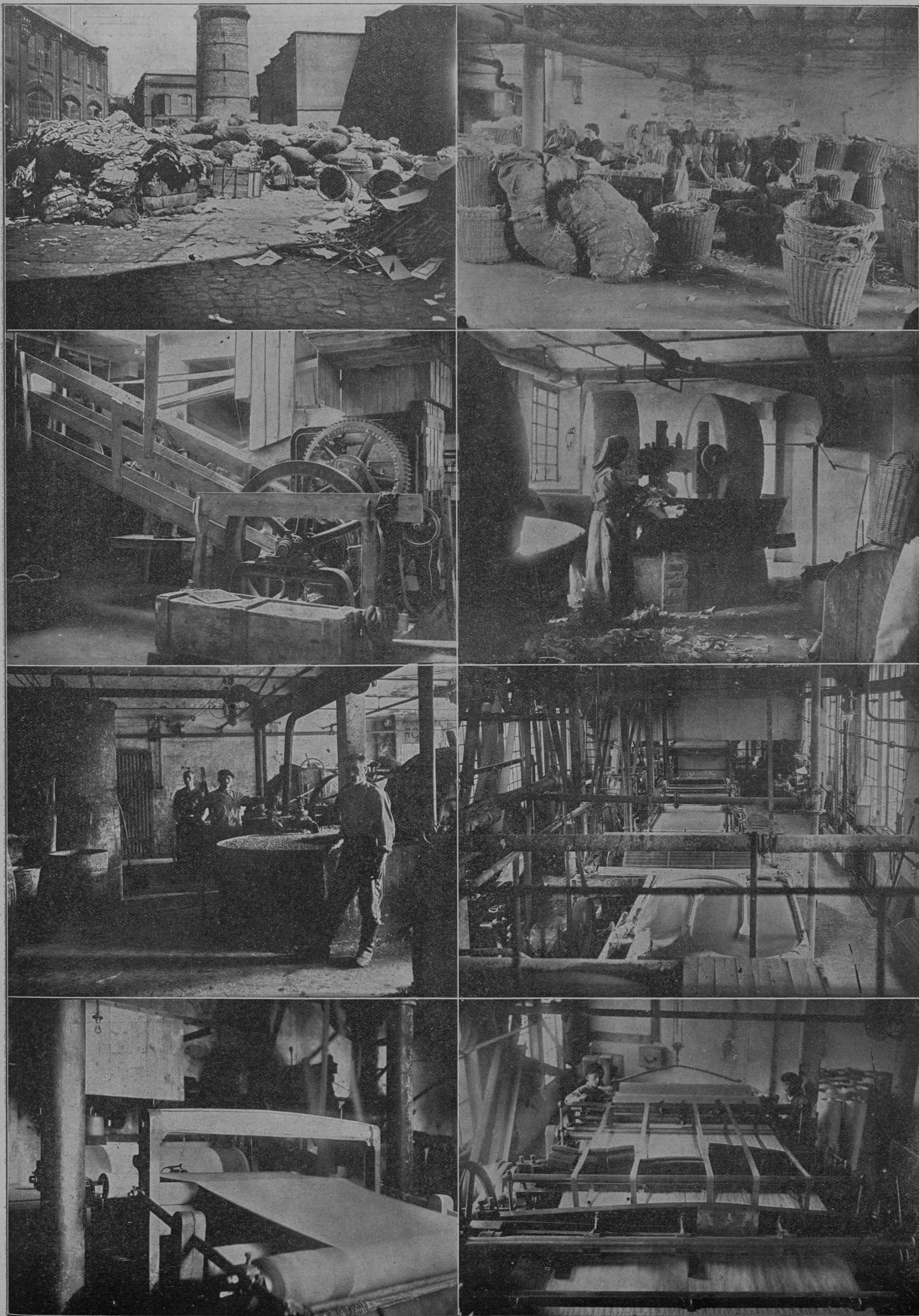
Izdelovanje papirja: Zgoraj: Na dvorišču papirnice grmade starega papirja lepenke in cunj. — Pripravljanje materiala. — Druga vrsta: Stroj za raztrganje cunj za papir. — Mlenje cunj — Tretja vrsta: Mešanje mase v čebrih. — Strojnica v papirnici. Spodaj: Zvijanje napolsuhega papirja. — Stroji režejo papir na razne velikosti in oblike.
