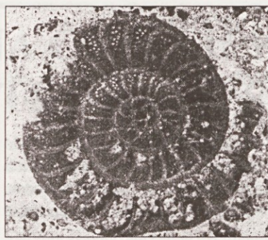
Prerez okrog 1 cm velike hišice luknjičarke Operculina exiliformis , ki je živel pred približno 54 milijoni let.
