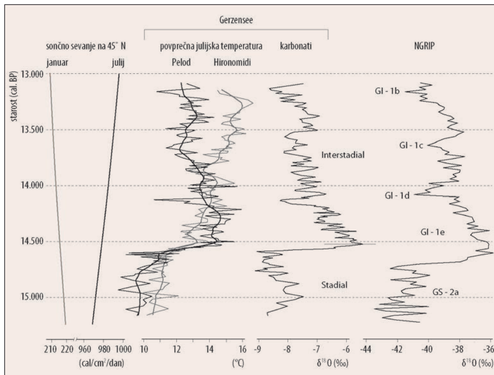
Sl. 133: Rekonstrukcija poznoglacialne temperature jezera Gerzensee na osnovi peloda, hironomidov in koncentracije kisikovih izotopov ( \delta^{18}\text{O} ). Rezultate primerjamo s količino sončnega sevanja na 45^\circ severne širine (prva krivulja) in razmerjem kisikovih izotopov ( \delta^{18}\text{O} ) v grenlandskem ledu vrtnice NGRIP (zadnja krivulja). Opazni sta dve hladni oscilaciji , ki so ju zaznali tudi na drugih najdiščih v srednji Evropi in v grenlandskem ledu (GI-1d in GI-1b). Po predlogi: Lotter s sod. 2012, sl. 4.
