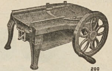
Br. 200: Stroj za rezanje šunke i salama, 3 veličine. Promj. oštrice mm 130 155 175 Cijena Din 720, 1200, 1900
