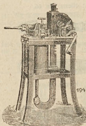
Br. 194: Stroj za punjenje kobasica, sistem Wien, sadržaj kg 5 8 13 20 Cijena Din 2400 2800 4800 5800.
