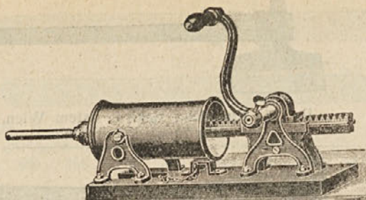
Br. 183: Stolni stroj za punjenje kobasica, sadržina 4 kg, cijena Din 650. Dobije se isti stroj sa gvožd. levanim kazanom od 5 kg sadržaja, cij. Din 850. Kazan kod ovog stroja je od limovine.
