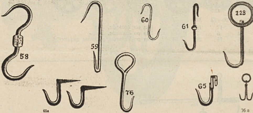
Br. 59 i 60: Pocin. S- ili pravokutno savita kuka mjera u mm 5×100 6×120 7×140 8×160 9×200 12×250 Cijena Din 2 3 4 5 6 8
