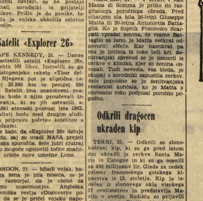
Satelit «Explorer 26»
