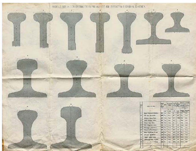
Profili železniških tračnic, ki so jih na Prevaljah izdelovali med letoma 1836 in 1852. (Deželni arhiv Celovec, AT-KLA, NL Rosthorn Franz)
