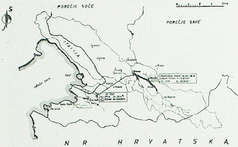
Situacijska skica hidroelektrarne Osp ali na kratko HC Koper
