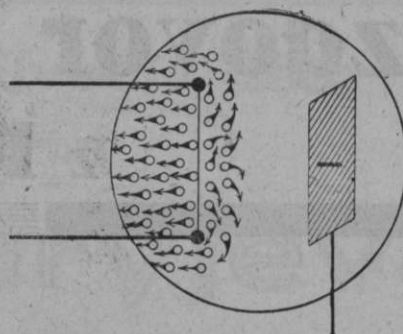
10. slika. Če se pomotoma naelektri elektronkina anoda negativno, odbija po nitki izžarjene elektrone in med nitko in anodo ni nobenega toka.
