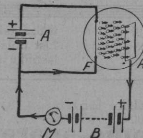
8. slika. Rišba kaže, kako sta zvezani nitka F in anoda A z baterijama A in B. Baterija A razžareva nitko F; B je anodna baterija. Tako se imenuje, ker je zvezana z anodo A. Galvanometer M kaže, ali teče v elektroniki tok od F proti A.
