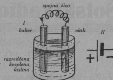
3. slika. I. Bakrena in cinkova palica v žvepleni kislini sestavljata galvanski člen. Elektroni se gibljejo v žici, ki veže obe palici, od cinka proti bakru. To gibanje elektronov imenujemo električni tok. — II. Poleg je narisana simbol člena, kakor ga rišemo v radio-tehniki.
