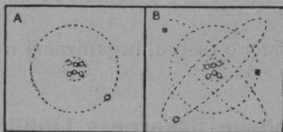
2. slika. Atom A je pozitiven, ker mu manjka en elektron; atom B je negativen, ker ima en elektron preveč.
