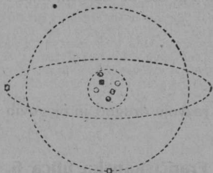
1. slika. Splošen ustroj atoma. V sredini je skupina štirih protonov, ki so označeni s 4 krogi, in dva elektrona, narisana kot kvadrata. Tako je sestavljeno atomovo jedro. Okrog jedra krožita v različnih razdaljah druga dva elektrona.
