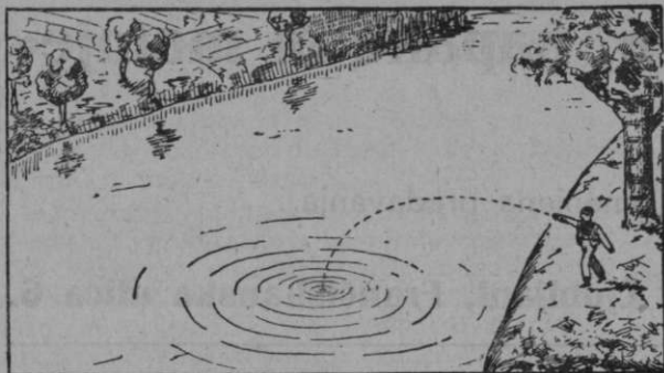
4. slika. Krožni valovi se razširjajo od mesta, kjer pade kamen v vodo. Sličen pojav nastane v etru, če ga moti nihanje elektronov.
