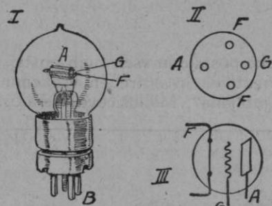
6. slika. I. Pregledna slika elektronke: A je anoda, G mreža, F nitka ali katoda, B so vtikala. Elektrode (anoda, mreža, nitka) so v stekleni posodici (večinoma v obliki valja), ki ima valjasto vznožje. Vznožje je iz izolatorja in je radi mehanske trdnosti včasih okovano. Vznožje nosi štiri vtikala, ki so navadno razvrščena, kakor kaže II. stranska slika. III. slika kaže simbol troelektrodne elektronke, kakor ga rišemo v stikalnih načrtih.
