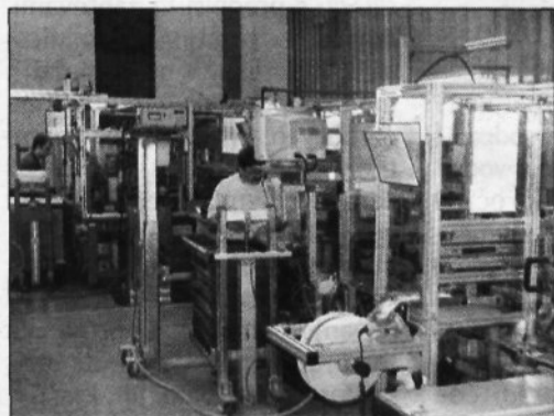
Avtomatske linije v Resistecovi proizvodnji v Krškem
