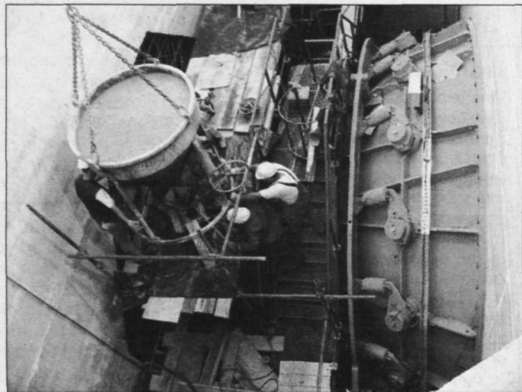
Na turbini v agregatu 3 potekajo še zaključna dela pred poskusnim zagonom.
