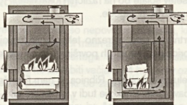
Kotel s pregorevanjem (levo) in kotel s spodnjim odgorevanjem
