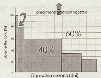
Obremenjenost kotla med ogrevalno sezono
