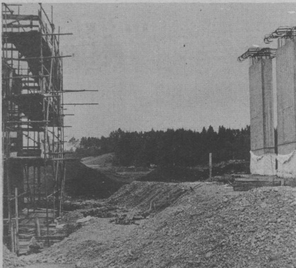
Graditev avtoceste Naklo—Ljubljana dobro napreduje
