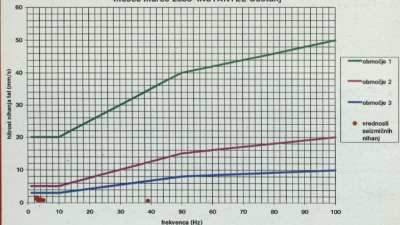
PRIMERJAVA ZABELEŽENIH NIHANJ TAL Z DOPUSTNIMI PO STANDARDU DIN 4150 ZA KRATKOTRAJNA TRESENJA ZA mesec marec 2005-INSTANTEL-Šoštanj
