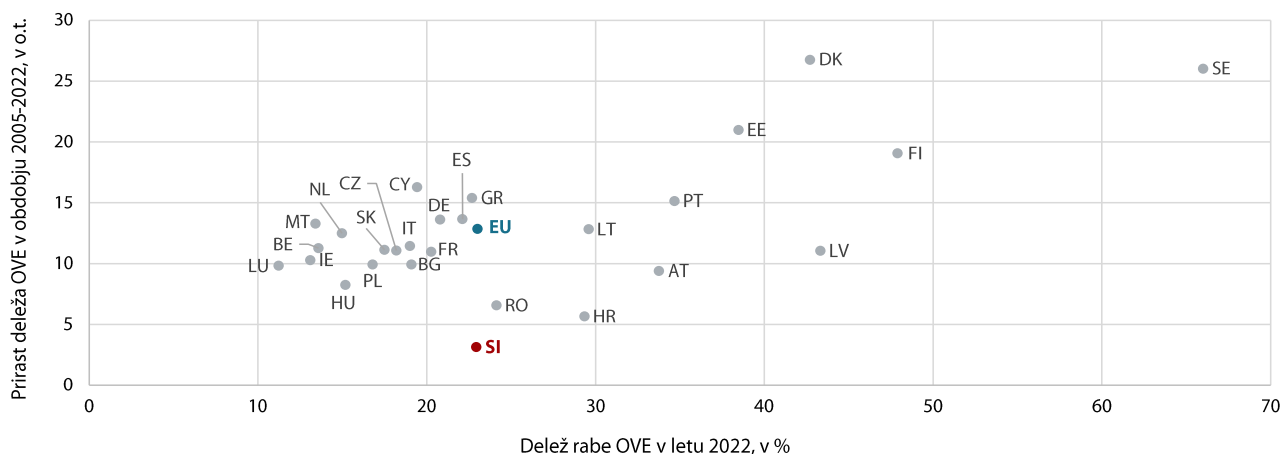
Slika: Delež rabe OVE* v letu 2022 ter povečanje deleža OVE v obdobju 2005–2022
