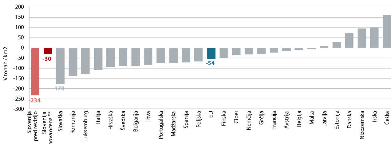
Slika: Ponori oz. izpusti TGP iz sektorja rabe zemljišč, spremembe rabe zemljišč in gozdarstva*, 2020
