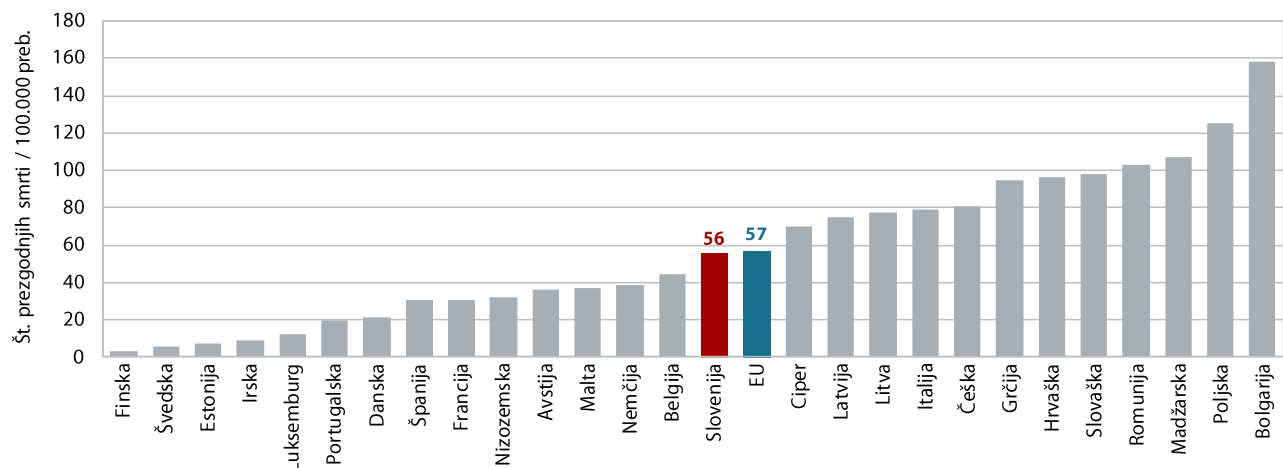
Slika: Prezgodnje smrti zaradi drobnih delcev PM 2,5 na 100.000 prebivalcev, 2021
