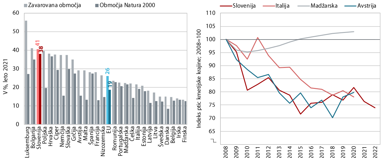
Slika 93: V Sloveniji je delež zavarovanih območij velik (levo), indeks ptic kmetijske krajine, ki je kazalnik sprememb biotske raznovrstnosti, pa je v zmernem upadu (desno)
