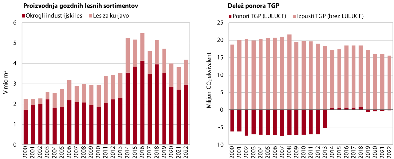
Slika 95: Proizvodnja gozdnih lesnih sortimentov, ki je bila v sanaciji gozdov po žledu (leto 2014) velika, se je zadnja leta zmanjšala, hkrati so se znižali tudi ponori toplogrednih plinov v gozdovih
