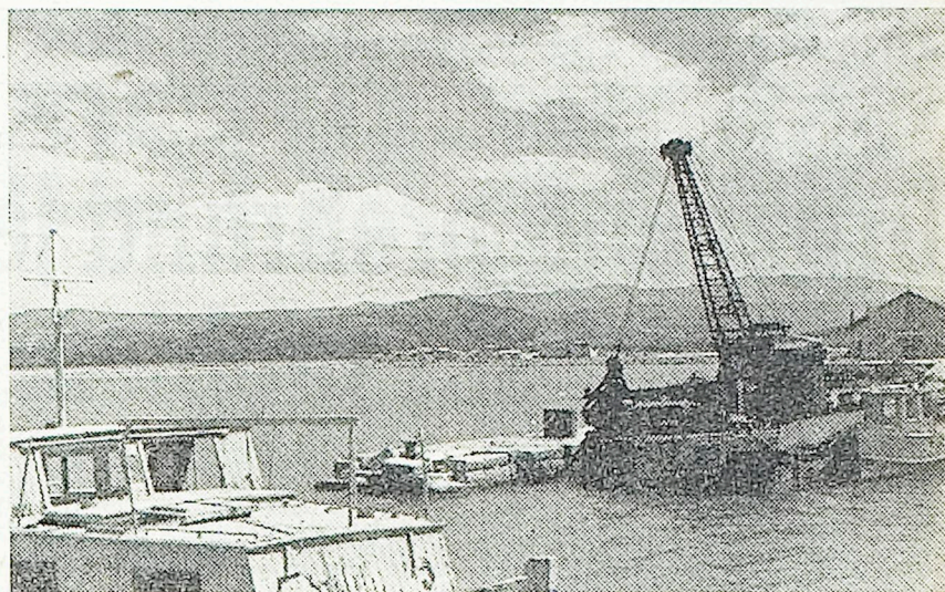
Od novega tovornega pristanišča se širi proti vzhodu širna planjava zasipane zaliva, kjer takoj za nasipom na prvih metrih osušenega zemljišča postavljajo temelje za nova skladišča lesa, ki bo šlo iz naše domovine ali v tranzitu prek Kopra po morski poti v širni svet. V ozadju je že videti rumene skladiščne deske, ki čakajo zdej še kar na prostem, da jih vkrajo na ladje in popeljejo kupcem v tujino
