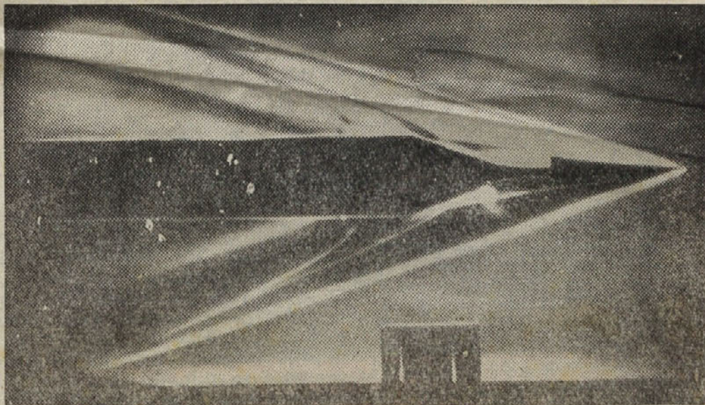
Pričujoča slika prikazuje zračne valove, ki nastajajo v poskusnem kanalu, ko veter z hitrostjo 6.500 km trči na koničasto oviro, podobno izstrelku. (AND)
