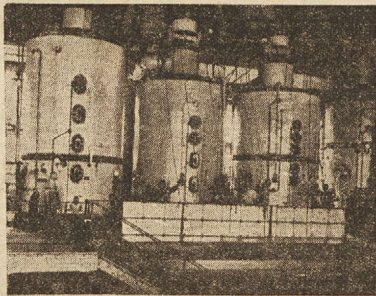
VAKUMSKI APARAT ZA PRIDELOVANJE SLADKORJA
