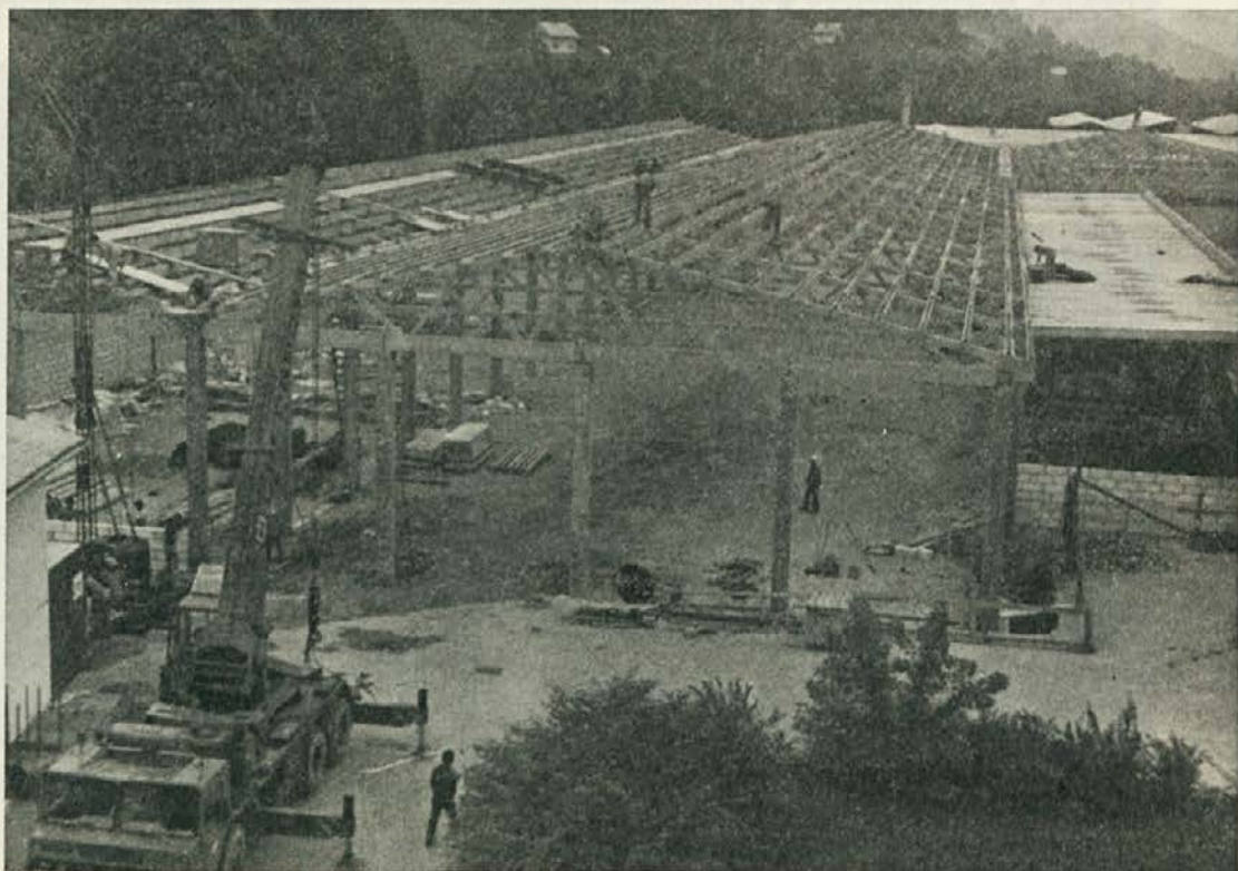
Betonska konstrukcija dobiva svojo obliko
