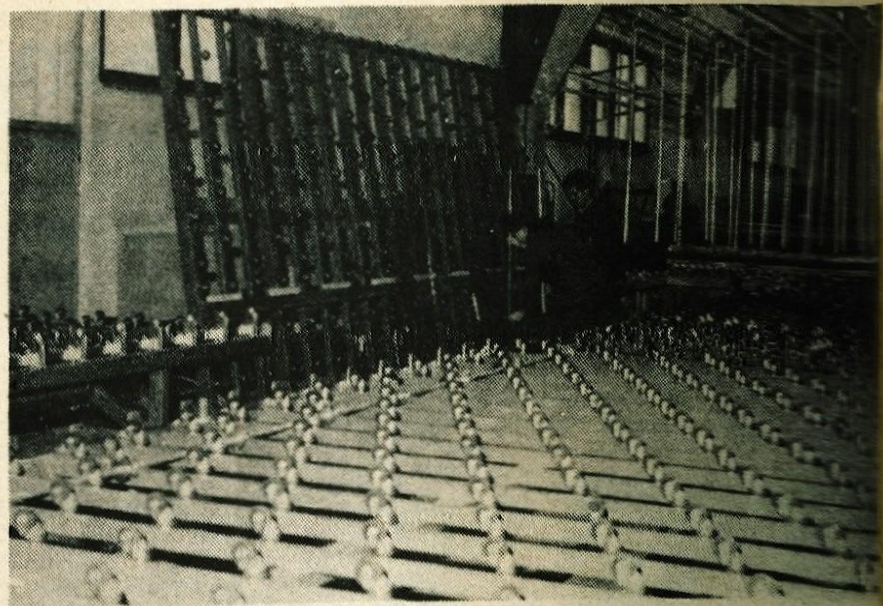
Proizvodnja izolacijskih stekel v tovarni na Trati.
