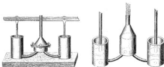
Ktesibilisova brizgalna
