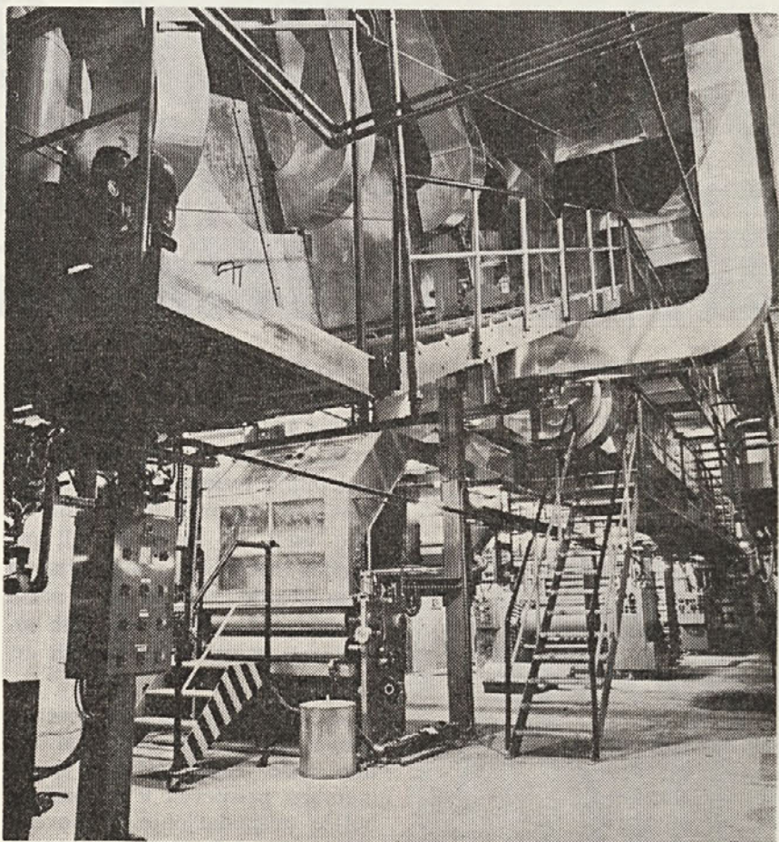
Premazovalni stroj S-3
