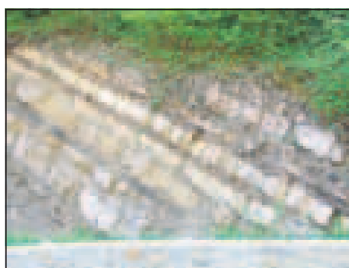
Strmški člen v dolini Pekel pri Borovnici
