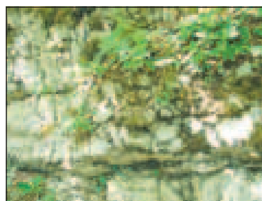
Plastnat apnenec ponekod razpada v diagenetsko brečo-konglomerat – Gredin apnenčev člen
