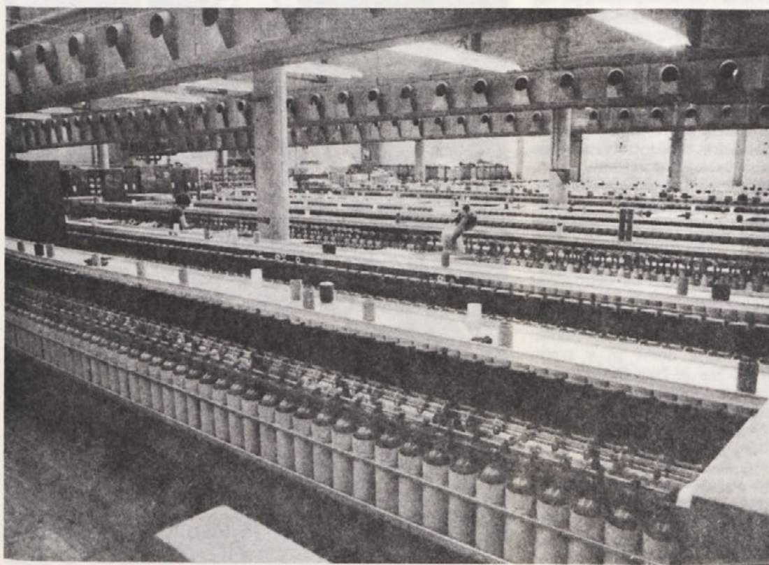
Sukanje na sodobnih sukalnih strojih (foto Pavlin).
