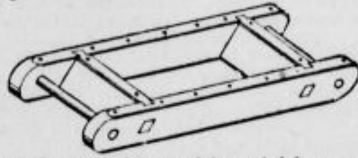
Sl. 2. Leseni kalup (model) za izdelavo opeke.
