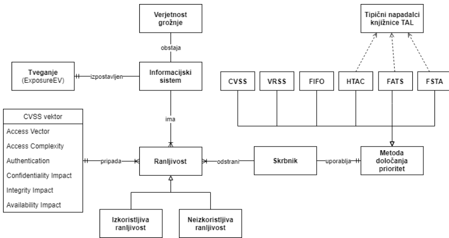
Slika 5.1. UML razredni diagram simulacijskega modela za merjenje učinkovitosti metod določanja prioriteta ranljivostim. S simulacijskim modelom preko spremenljivke ExposureEV k merimo izpostavljenost IS grožnjam, tj. izkoristljivim ranljivostim.
