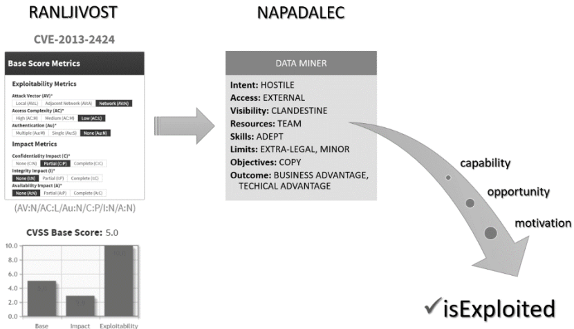
Slika 4.1. Funkcija izkoriščanja isExploited se ovrednoti tako, da napadalec primerja svoje lastnosti z lastnostmi ranljivosti. Če je dovolj sposoben ( capability ) in motiviran ( motivation ) in če opisana ranljivost zanj predstavlja priložnost ( opportunity ), je zmožen izkoriščanja. Ranljivost je predstavljena s CVSS vektorjem, napadalec pa z atributi knjižnice TAL.
