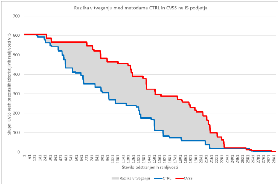
Slika 7.4. Graf prikazuje razliko v tveganju pri uporabi metod CTRL in CVSS na IS podjetja. Učinkovitejša metoda hitreje zmanjšuje tveganje (nižja vrednost kazalnika RiskMitigation k ).
