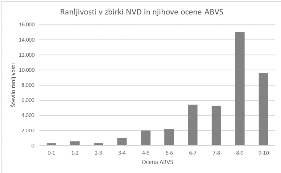
Slika 6.8. Porazdelitev ocen ABVS ranljivosti v zbirki NVD.
