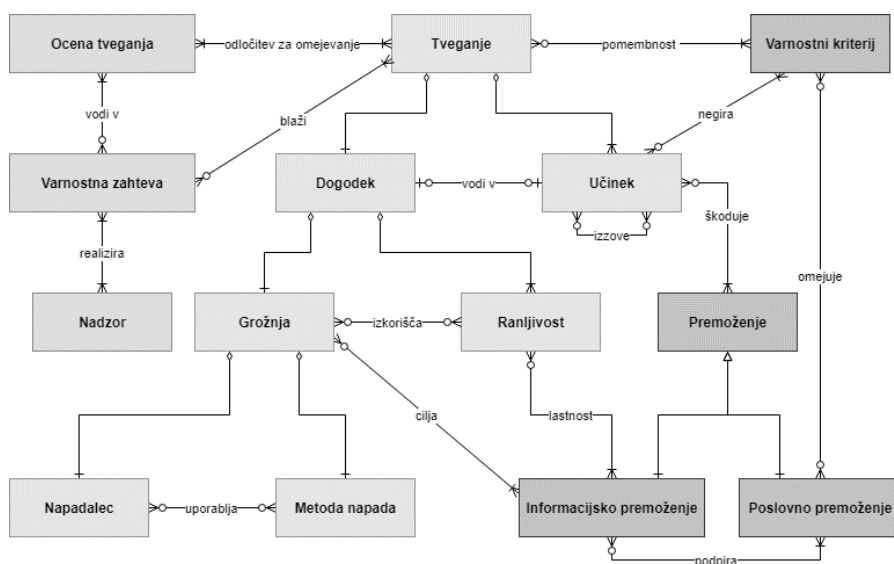
Slika 2.7. Predstavitev področja varnostnih tveganj v IS z UML razrednim diagramom (angl. Information System Security Risk Management domain model, ISSRM ) (Dubois idr., 2010, str. 12).
