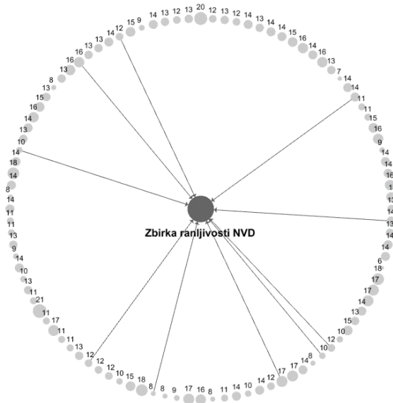
Slika 6.1. Simulacijski model za izračun frekvenc izkoriščanja vektorjev CVSS v podatkovni zbirki NVD med izvajanjem. V središču je informacijski sistem, ki vsebuje vse ranljivosti zbirke NVD od leta 2010 do leta 2016. Okrog sistema so naključno ustvarjeni napadalci, predstavljeni z različno velikimi pikami. Velikost pike je odvisna od vrednosti napadalčevih atributov (vsota vrednosti urejenostnih atributov). Večja pika predstavlja napadalca z močnejšimi atributi oz. večjo grožnjo. Puščica v smeri od napadalca k sistemu pove, da je napadalec zmožen izkoristiti naključno najdeno ranljivost v NVD.
