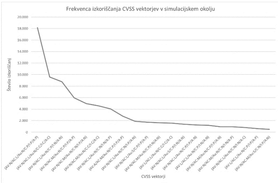
Slika 6.3. Frekvence izkoriščanja vektorjev CVSS v simulacijskem okolju. Na sliki je prikazanih 20 najpogosteje izkoriščanih vektorjev. Vrednosti so urejene od najvišje do najnižje. Z grafa lahko razberemo, da frekvenca pada eksponentno. Mnogi vektorji CVSS niso nikoli izkoriščeni.
