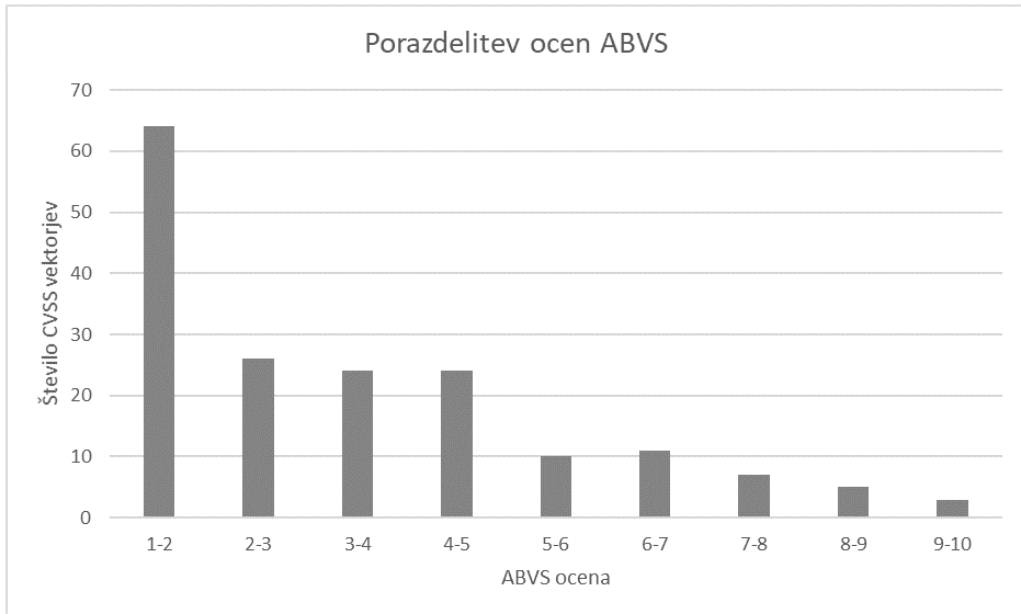
Slika 6.7. Porazdelitev ocen ABVS za vektorje CVSS, ki imajo frekvenco izkoriščanja večjo od 0.
