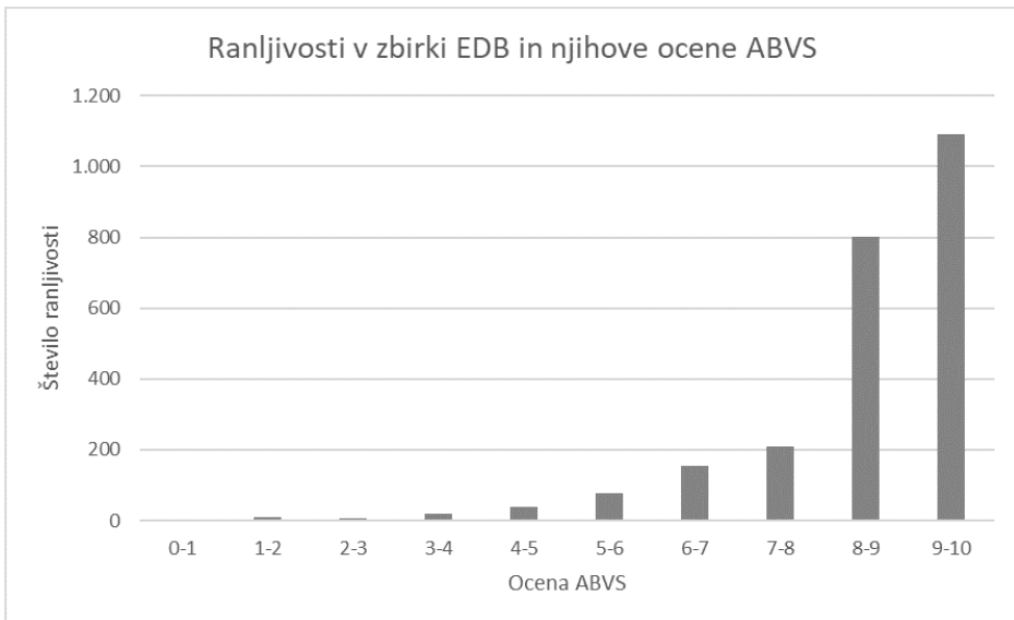
Slika 6.9. Porazdelitev ocen ABVS ranljivosti v zbirki EDB. Za ranljivosti v tej zbirki obstajajo koncepti izkoriščanja (angl. Proof of Concept Exploits ).
