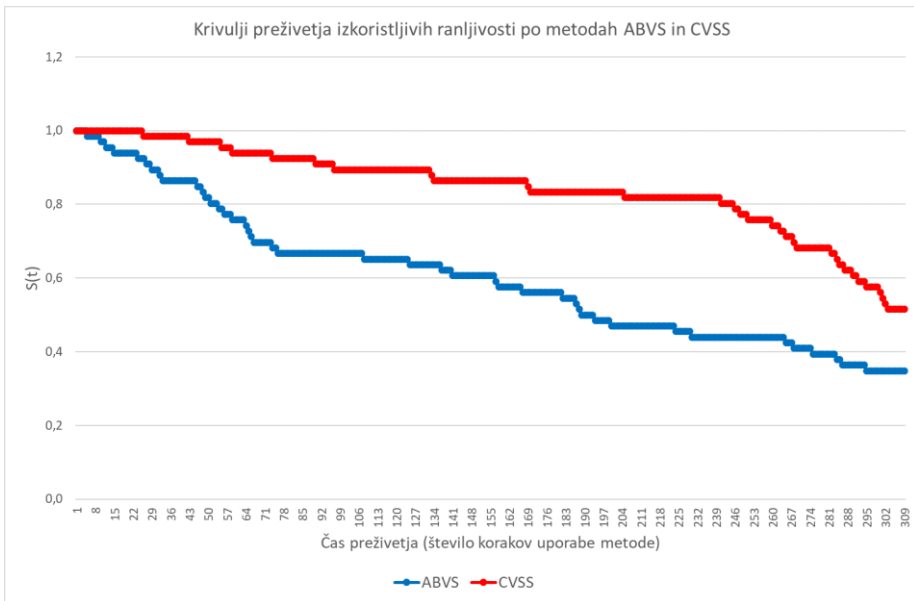
Slika 6.6. Slika prikazuje krivulji preživetja metod ABVS in CVSS na eni izmed simulacij. Čas predstavlja zaporedni korak odstranjevanja ranljivosti.
