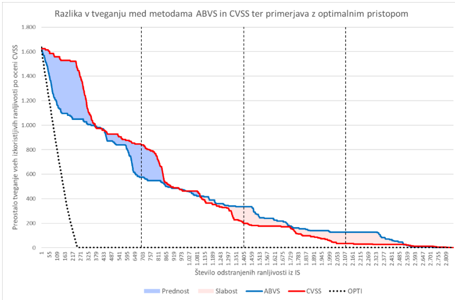
Slika 7.2. Graf prikazuje razliko v tveganju pri uporabi metod ABVS in CVSS na IS za spletno gostovanje. Tveganje je merjeno z ocenami CVSS preostalih izkoristljivih ranljivosti v IS. V prvem delu metoda ABVS hitreje zmanjšuje tveganje. V drugem delu je boljša metoda CVSS. Po kazalniku RiskMitigation k je v celoti gledano učinkovitejša tista metoda, pri kateri je preostalo tveganje manjše (razlika označenih površin na grafikonu). Krivulja OPTI predstavlja idealen pristop pri odstranjevanju ranljivosti.
