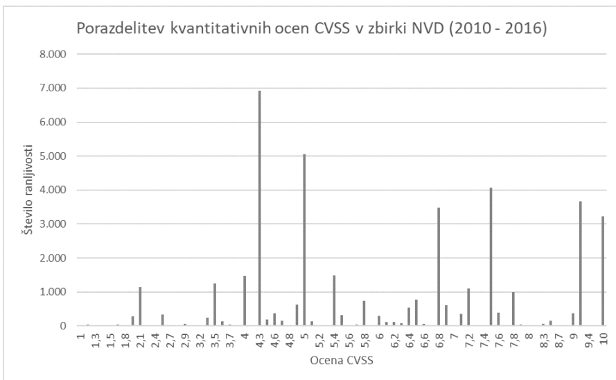
Slika 3.5. Porazdelitev kvantitativnih ocen CVSS ranljivosti v podatkovni zbirki NVD v obdobju 2010 – 2016.
