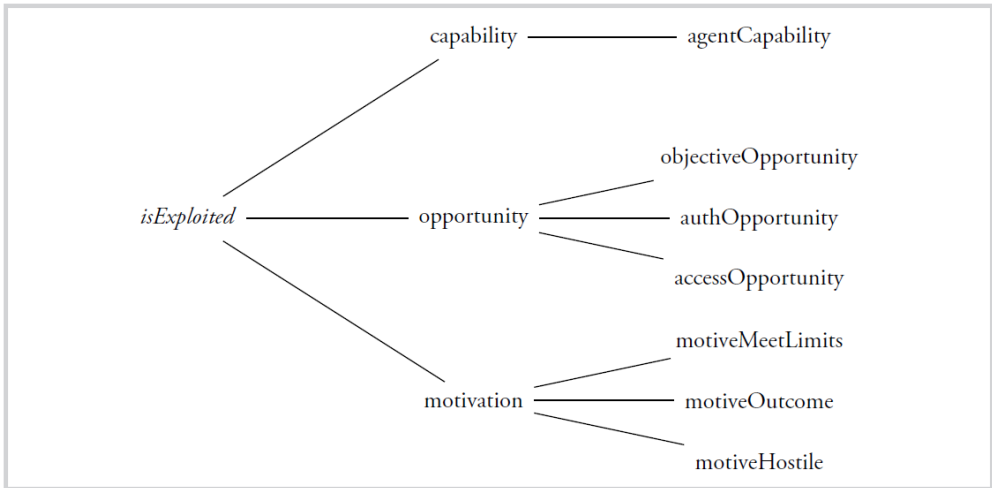
Slika 4.4. Diagram povezav vseh opredeljenih spremenljivk pri ovrednotenju funkcije izkoriščanja ranljivosti isExploited .
