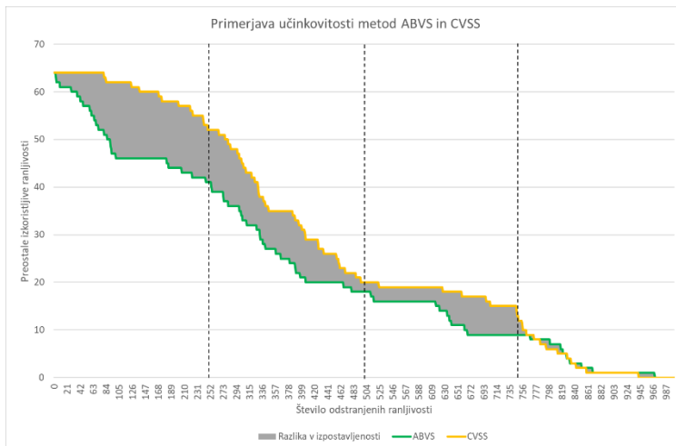
Slika 6.5. Primerjava učinkovitosti metod ABVS in CVSS. Površina med krivuljama pokaže, za koliko je metoda ABVS uspešnejša pri odstranjevanju izkoristljivih ranljivosti oz. pri omejevanju izpostavljenosti IS grožnjam.
