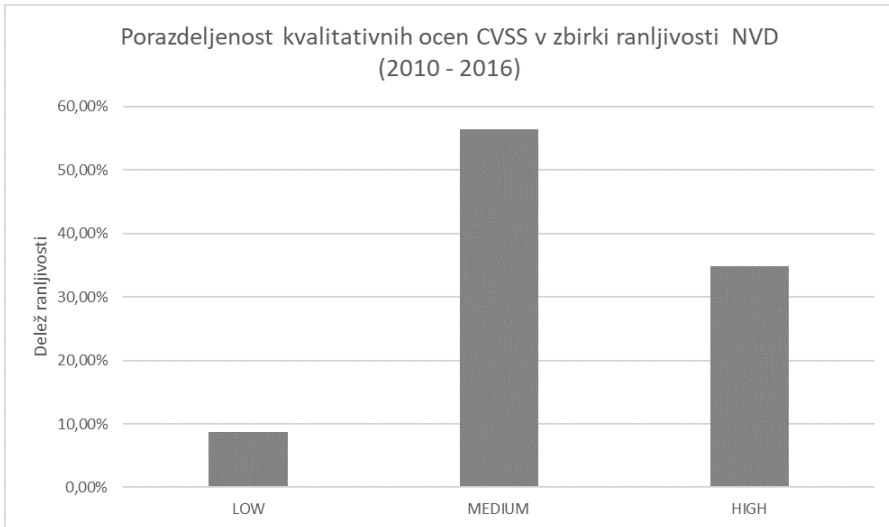
Slika 3.6. Porazdelitev kvalitativnih ocen CVSS v podatkovni zbirki NVD v obdobju 2010 - 2016.
