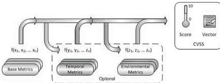
Slika 3.3. Postopek izračuna ocen CVSS. Ocena CVSS Base vedno obstaja in je na voljo v zbirki NVD. CVSS Temporal se izračuna na osnovi ocene CVSS Base, CVSS Environmental pa na osnovi ocene CVSS Temporal (Mell idr., 2007, str. 5).
