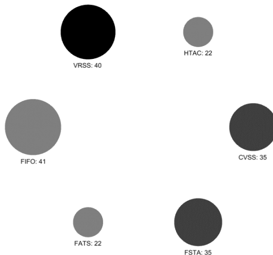
Slika 5.3. Primerjava učinkovitosti metod v simulacijskem okolju. Poleg imena vsake metode je navedeno število preostalih izkoristljivih ranljivosti v informacijskem sistemu. Učinkovitejša metoda hitreje odstranjuje izkoristljive ranljivosti.
