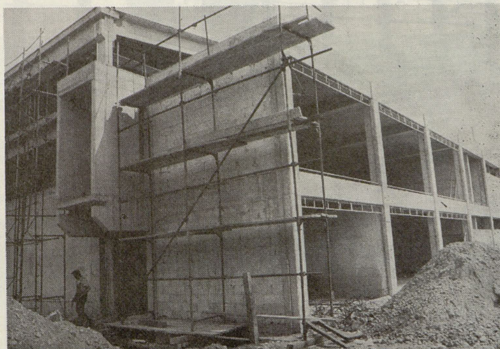
Gradnja
