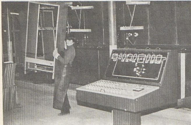
Obnovljena in posodobljena lužilnica v obratu Zamrzovalne omare.
