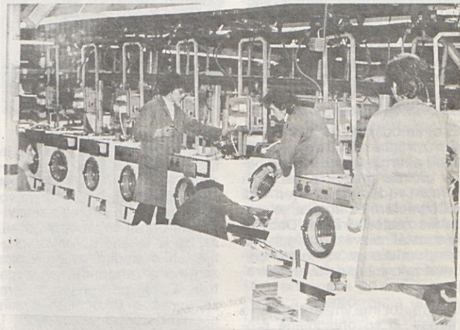
Prvi pralni stroji s 1000 obrati v redni proizvodnji
