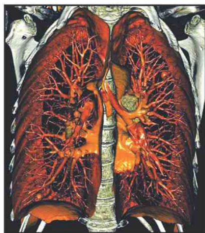
CT pljuč
