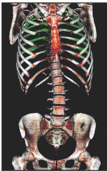
CT skeleta
