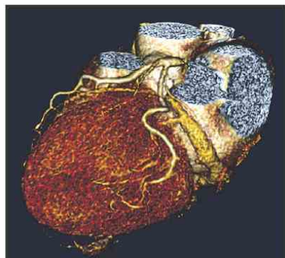
CT srca
