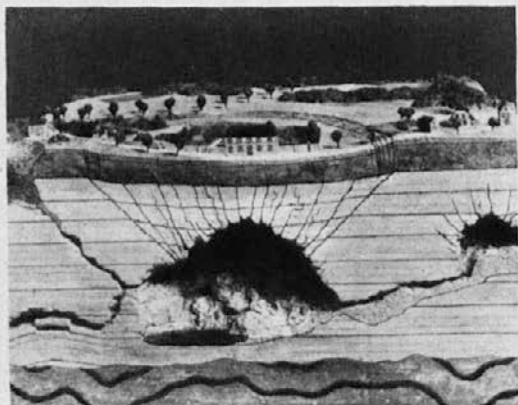
Kako deluje potres (po prof. Sieburgu)
