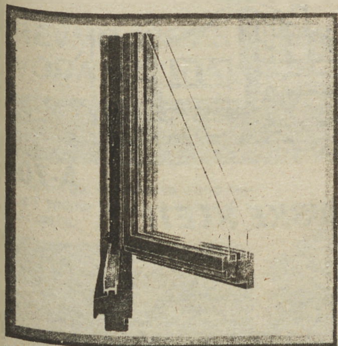
VEZANO OKNO — PREREZ
