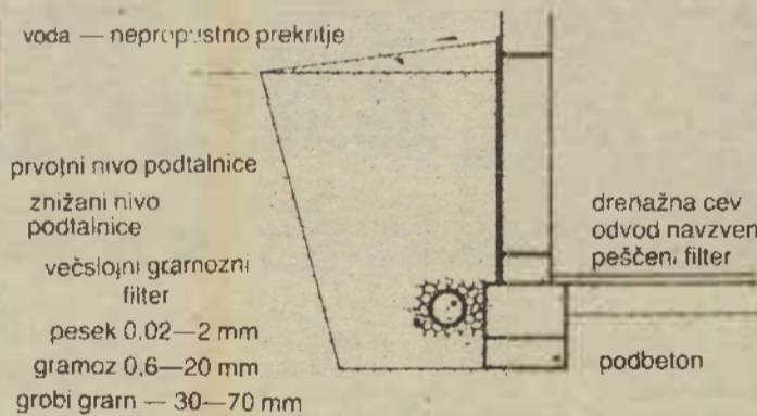
Sl. 2, primer pravilne izvedbe drenaže pri podkletenih zgradbah.
