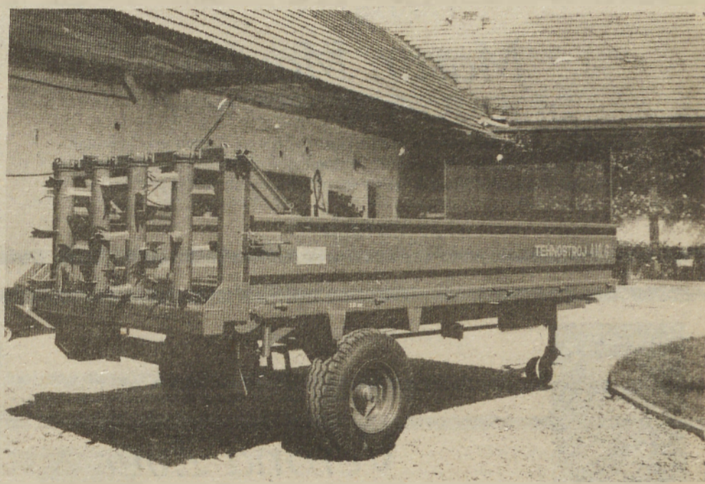
Trosilec hlevskega gnoja tip TEHNOSTROJ 411.6, nos. 4 tone, ima trosilno napravo s pokončnimi valji, kateri omogočajo enakomerno trošenje gnoja od 4 do 6 m. Trosilec je izdelan v izboljšani izvedbi iz visokokvalitetnih materialov, kateri mu dajo dolgo dobo uporabnosti. Z demontažo trosilne naprave dobimo enostavno prikolico. Z montažo poviškov stranic povečamo zaboj prostornino in trosilec lahko uporabljamo za prevoz silaže, sladkorne pese, krompirja in podobno. Zaboj se prazni s pomočjo transportnega traku, ki je na podu trosilca.
