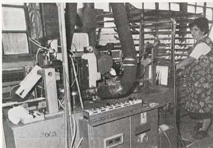
Rezkanje stranskega profila smuči
